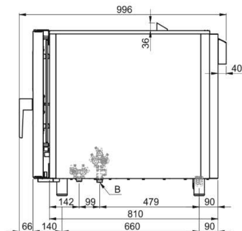
Vue côté
