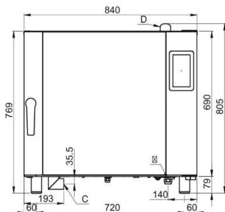
Vue face
