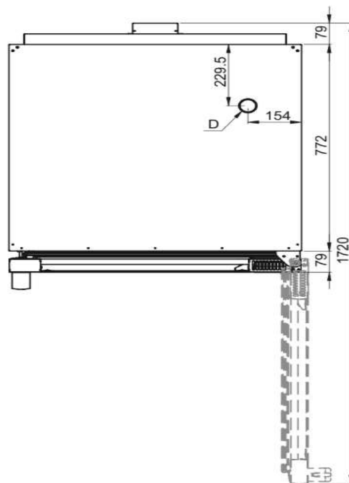
Vue de haut porte ouverte
